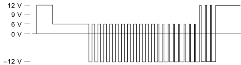
Figura A.6 – Secuencia de ensayo utilizando un circuito piloto de control simplificado
