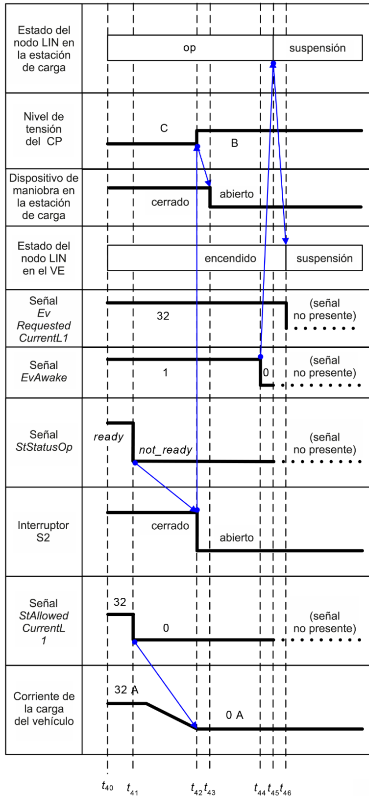
Figura D.6 – Ejemplo de cronograma para parada normal de la carga activada por la estación de carga
