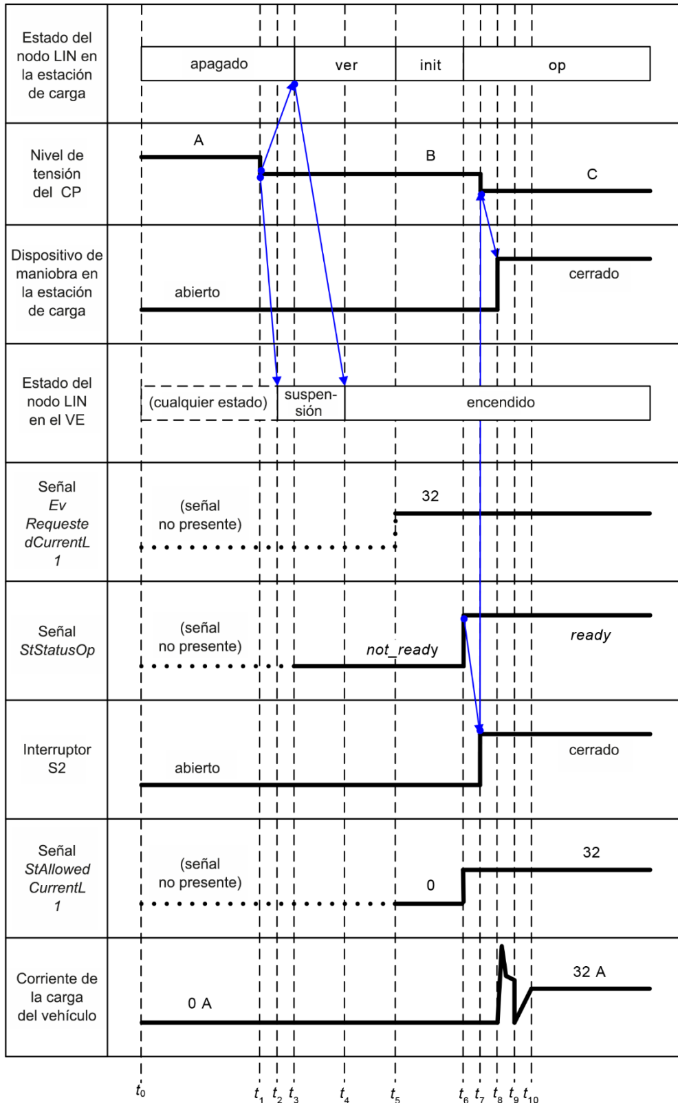
Figura D.4 – Ejemplo del cronograma para la puesta en marcha de la secuencia de carga normal en c.a.
