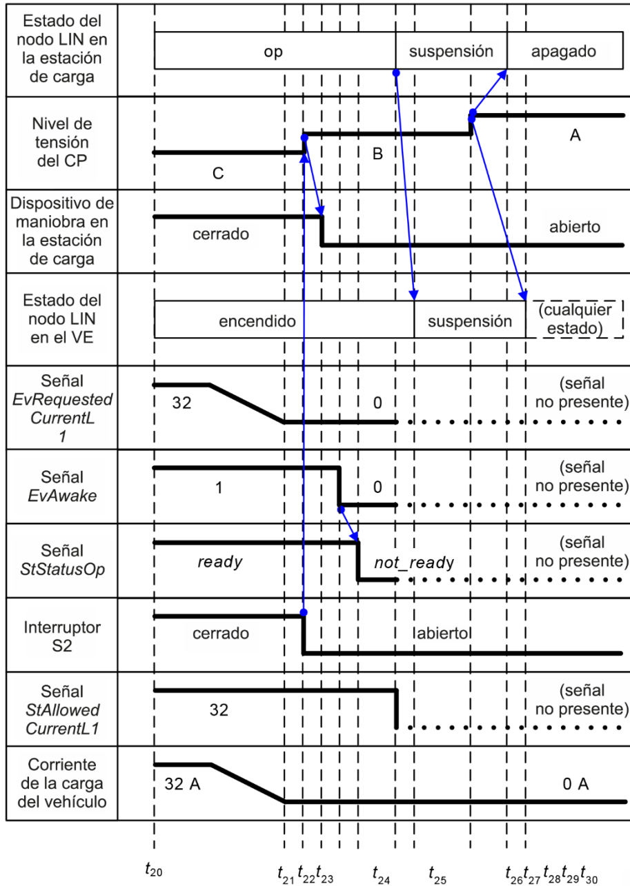
Figura D.5 - Cronograma para parada normal de carga activada por el VE
